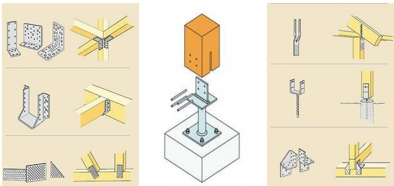
Зураг 6. Саравч, сүүдрэвчийн хэсэглэлийн холбоос, бэхэлгээ /жишээ/
