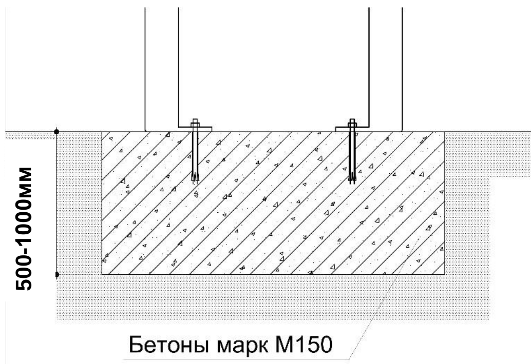
Зураг 12. Саравч, сүүдрэвч суурилуулах хэсэглэл
